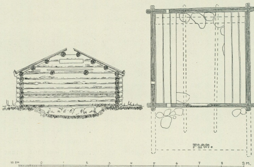
Fig. 41. Eldhus. Tvärsnitt och plan. Asplok. Samma som fig. 24.
