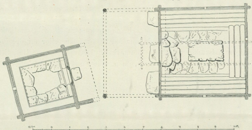
Fig. 22. Eldhuset fig. 21 jämte mjölkstuga.
