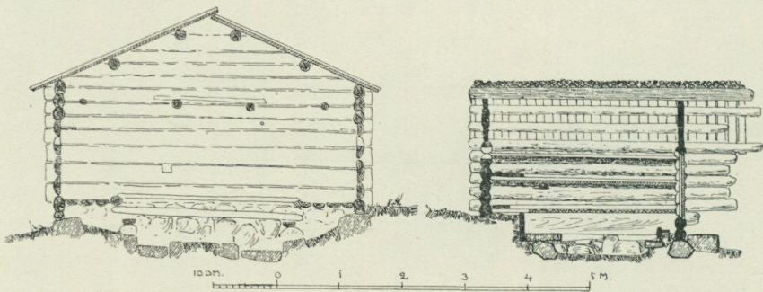
Fig. 43. Eldhus. Tvärsnitt. Mjölkstuga. Längdsnitt. Hedbodarna. Samma som fig. 21, 22.
