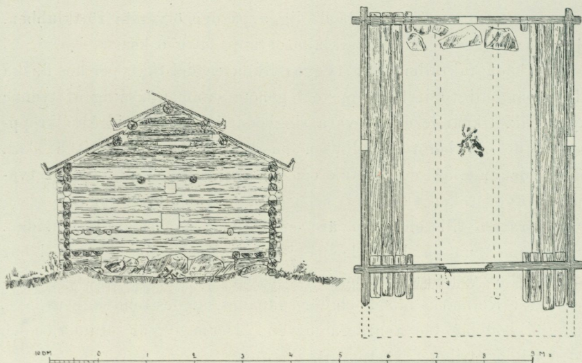
Fig. 40. Eldhus. Tvärsnitt och plan. Yttre Navardalen, Älfdalen, Dalarna. Samma som fig. 26.
