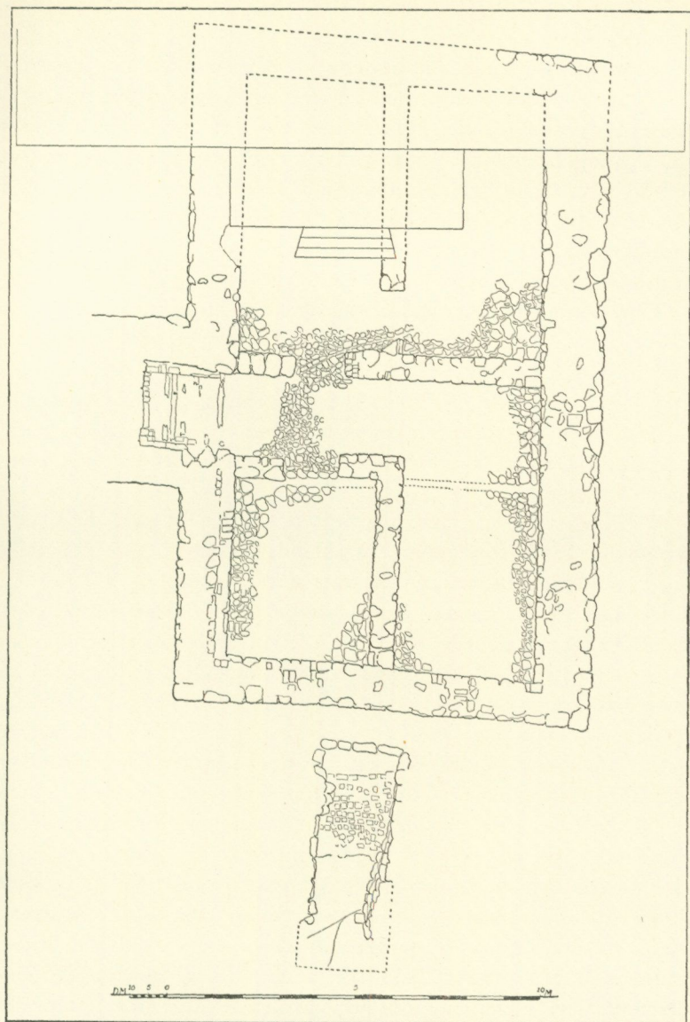
Bild 2. Stengrunden. Uppmätningsskizzen med konturen av »Prinsvillans» sydöstra fasad markerad genom heldragen, fin linje.
