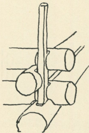
Fig. 4. Stenkistans hörnkonstruktion.
