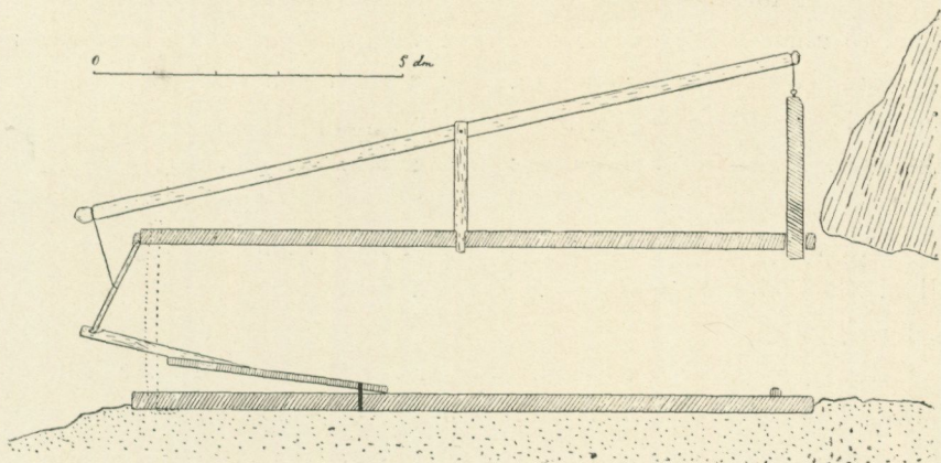
Fig. 2. Gräflingsfälla, uppgillrad. Längdgenomskärning. Grenna socken.
