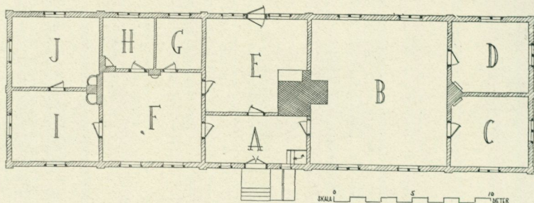
Fig. 4. Plan av herrgårdsbyggnaden från Hallstahammar.
