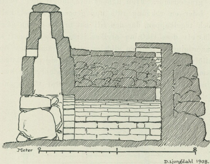
Fig. 2. Bastu vid Backa, Vaddö, Uppland. Längdsnitt.
