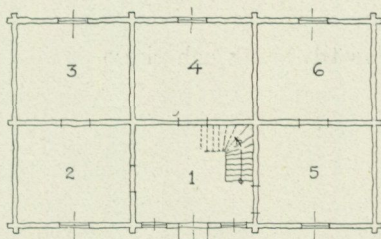
Fig. 26. Plan av boden. 1. Förstuga med jordgolv och två smala fönster, våg och trappa. 2. »Brännvinsbod». Gubben Ullholms sanctum sanitore. Dörren låstes med hänglås och dörrnyckel. 3 och 4. Mjöl- och varurum. 5. Visthus med silltunnor m. m. 6. Köttbod med galler för gluggen och lucka. Stengolv. — Alla dörrar i denna byggnad hade »kathål».
