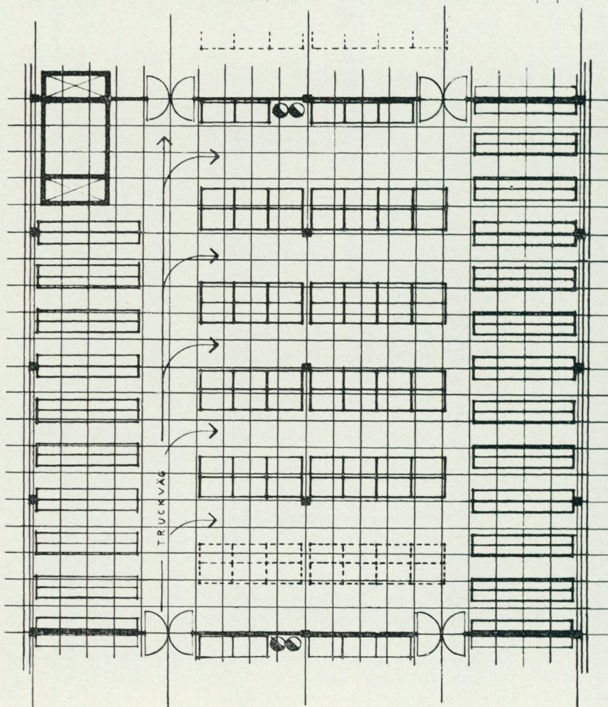
6. Sektion och plan av enhet för före- målsförvaring.
