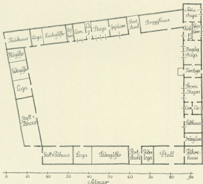
Fig. 4. Hemmesdynges prästgård, plan 1720.
