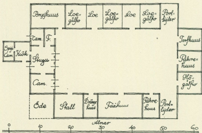
Fig. 3. V. Hoby prästgård, plan 1710.
