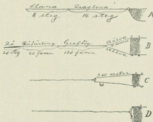
Fig. 26. Not-gen med draginrättningar af olika typer. (De olika delarnas längd är af utrymmesskal ej proportionellt återgifven å skisserna.) A Hornborga, Vgld. B Harön, Stockholms skärgård. C Mangskog, Vmld. D Skedevi, Ögld.
