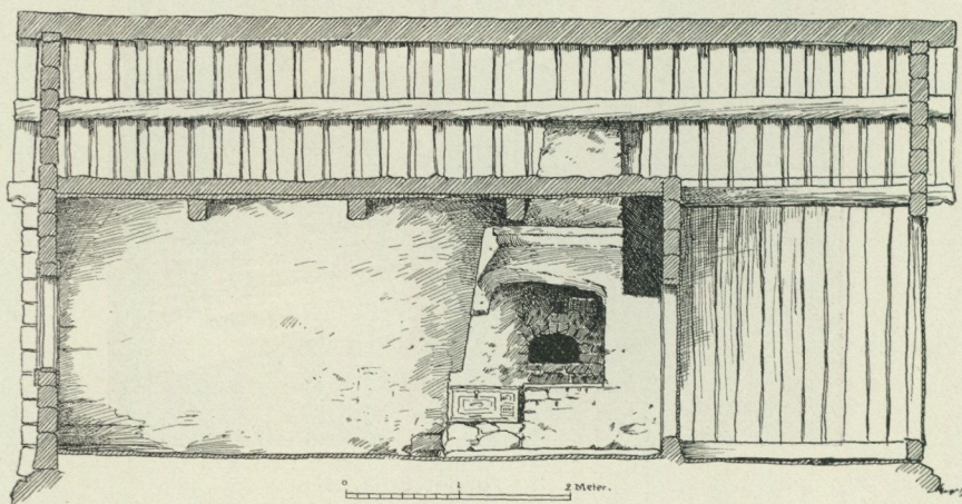
Fig. 3. Längdsnitt af torpet Sola.
