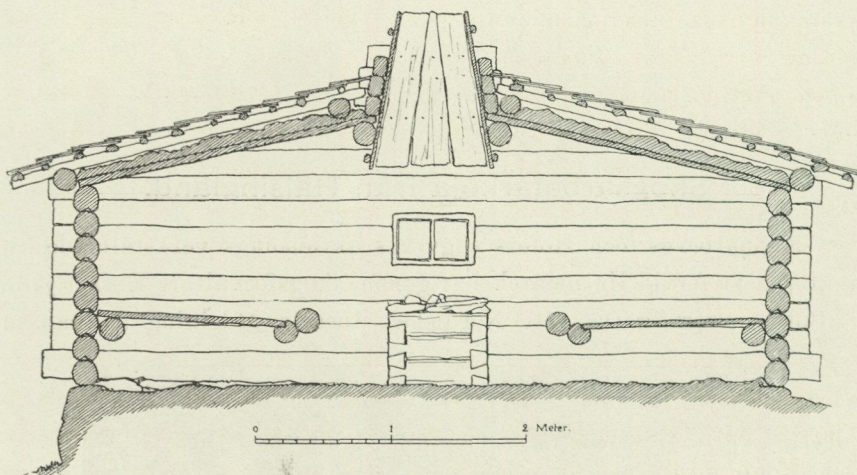
Fig. 2. Tvärsnitt af skogsarbetarkojan.
