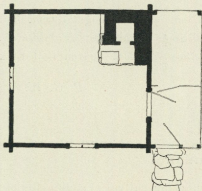
Fig. 2. Plan af torpet Sola.
