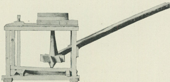
Fig. 10. Fotkvarn. Leksak från Värmland. H. 420 mm.
