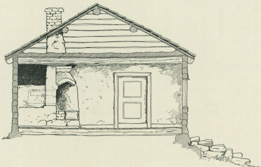
Fig. 4. Tvärsnitt af torpet Sola.
