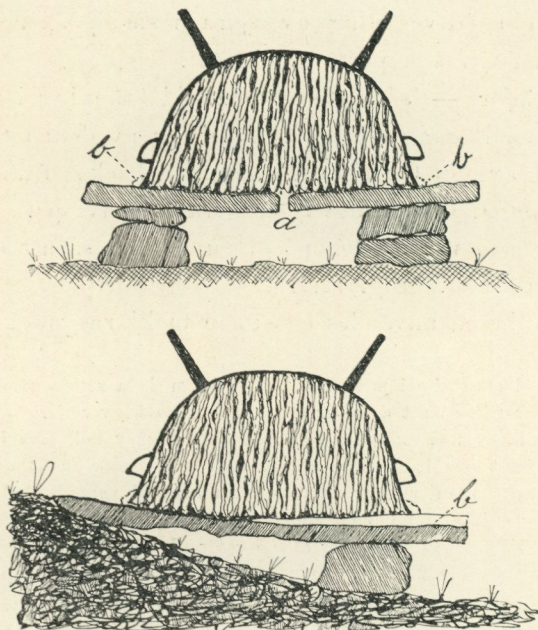
Fig. 12, 13. Tjärgrytor, fyllda med töre. Tvärsnitt. I övre bilden utgöres avloppet av ett hål, a , mitt i hallen; i den undre av en huggen ränna, b , som löper ut till hallens kant. Brunskog.
