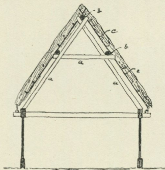
Fig. 7. Tvärsnitt av ett agtäckthus. Efter K. A. Berlin. Ur Arkitektur 1920.
