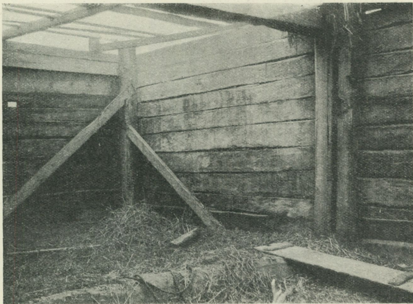
Fig. 5. Lada, Biskops, Gränsen mellan den äldsta delen och den yngre förlängningen åt väster. Förf. fot. 1909.
