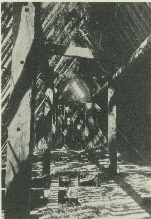
Fig. 8. Lada, Biskops. Interiör från vinden sedan ena takfallets agtäckning avlägsnats. Förf. fot. 1909.
