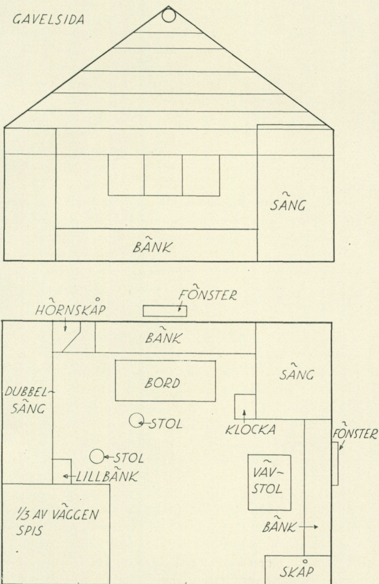
Bild 3—4. Tvärsnitt och plan från Örjangården, Bengtsarvet, Sollerö socken, Dalarna. Efter skiss av Artur Hazelius 1875.
