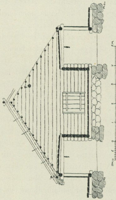
Fig. 24. Tvärgenomskäring af sjöboden fig. 14 och 35. Marviken, Vaddö.
